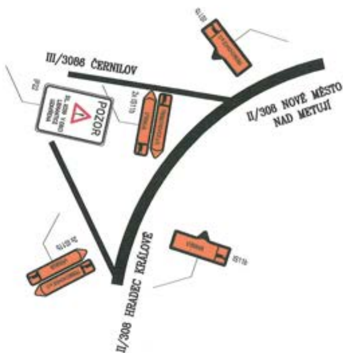
DETAIL 23.
