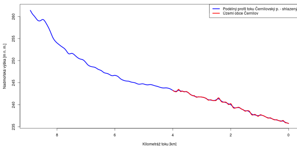
Obrázek 4: Podélný sklon vodního toku Černilovský potok
